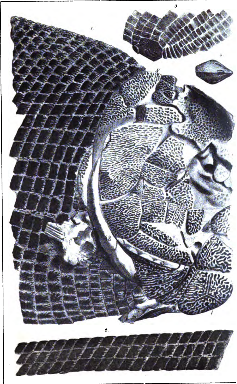
Quenstedt's Fossil.
